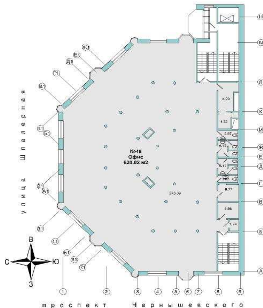
План 2 этажа
